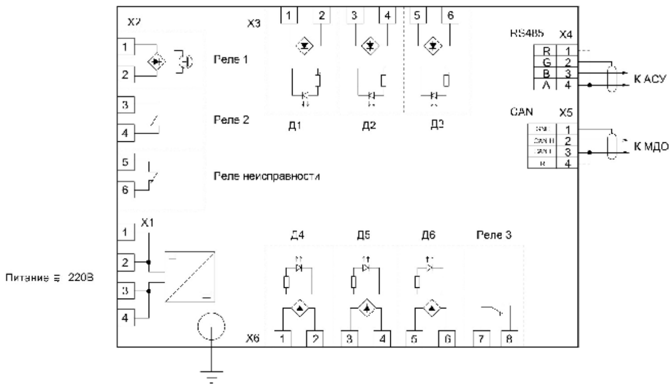
Рисунок В.2 – Схема подключения ТЭЗ-24
