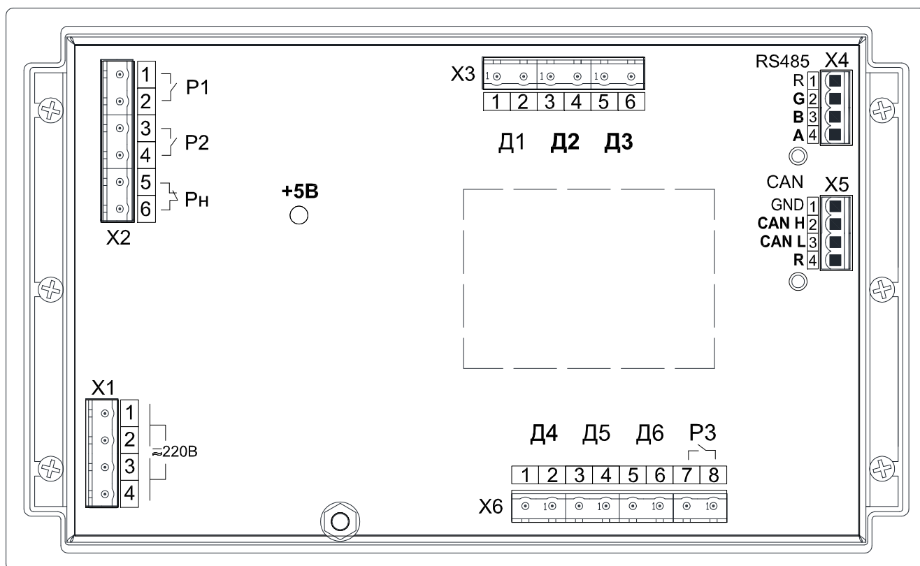
Рисунок Б.1 – Вид задней панели ТЭЗ-24
