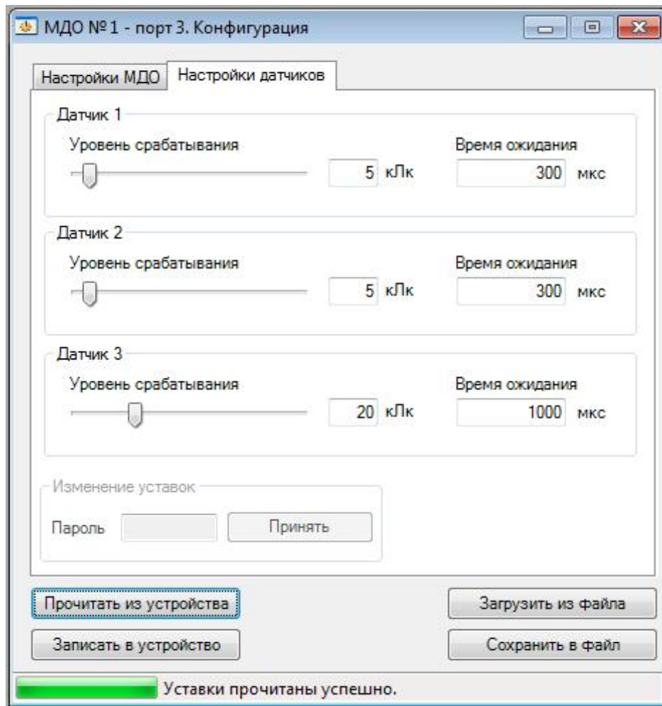
Рисунок 5.6 – Окно конфигурации МДО-1 «Настройки датчиков»
