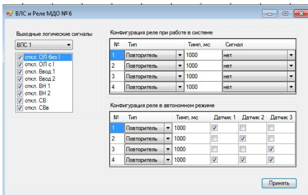
Рисунок 6.5 – Окно конфигурации выходных логических сигналов и реле МДО-1 «ВЛС и Реле МДО № ...»
