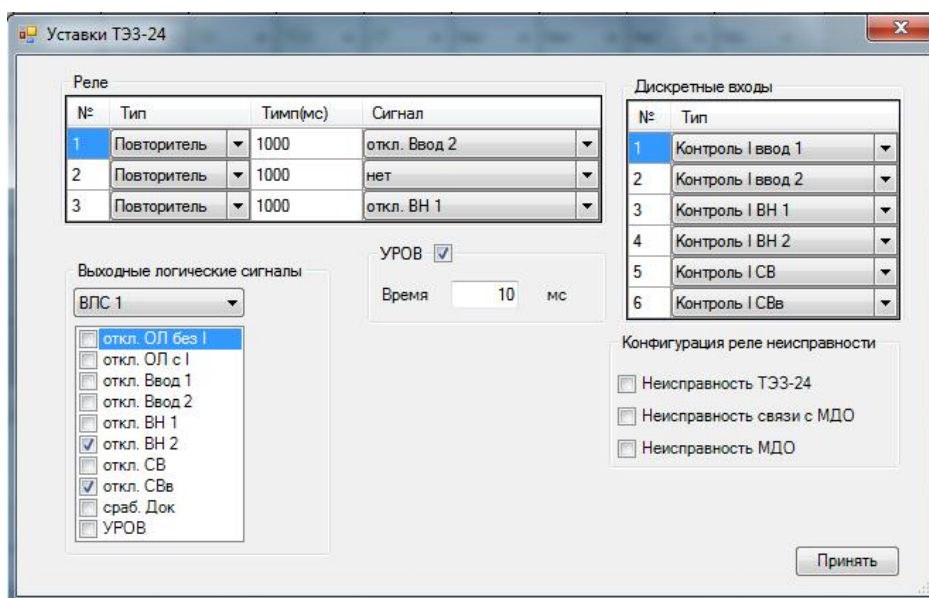
Рисунок 6.6 – Окно конфигурации ТЭЗ-24 «Уставки ТЭЗ-24»
