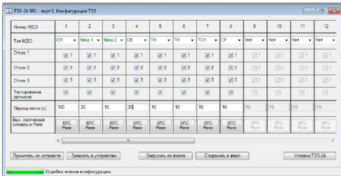
Рисунок 6.4 – Окно конфигурации ТЭЗ-24
