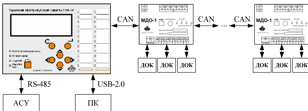
Рисунок 3.1 – Структура системы
