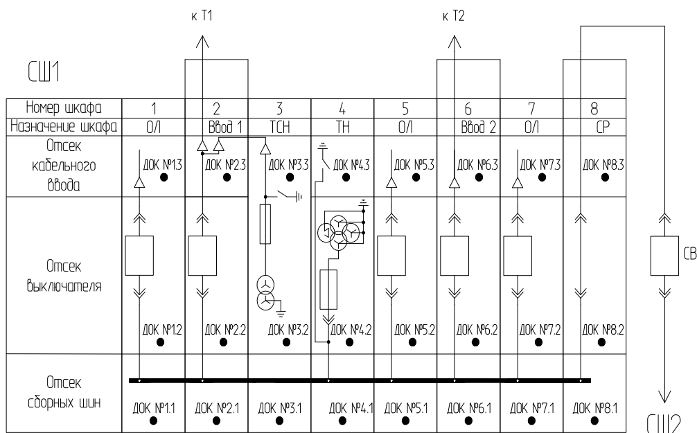
Рисунок 3.7 – Пример расположения ДОКов в шкафах
