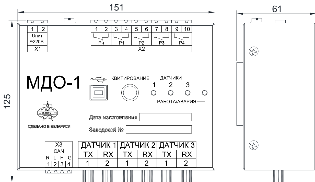
Рисунок А.1 – Габаритные размеры МДО-1 (без ДОК)
