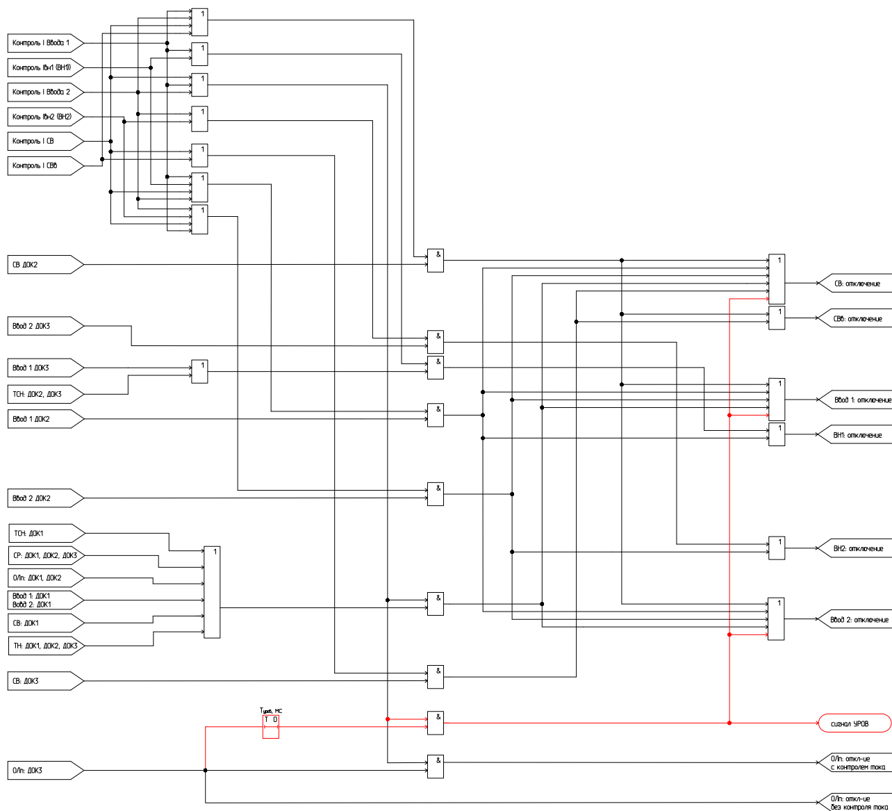
Рисунок 3.8 – Логика работы ТЭЗ
