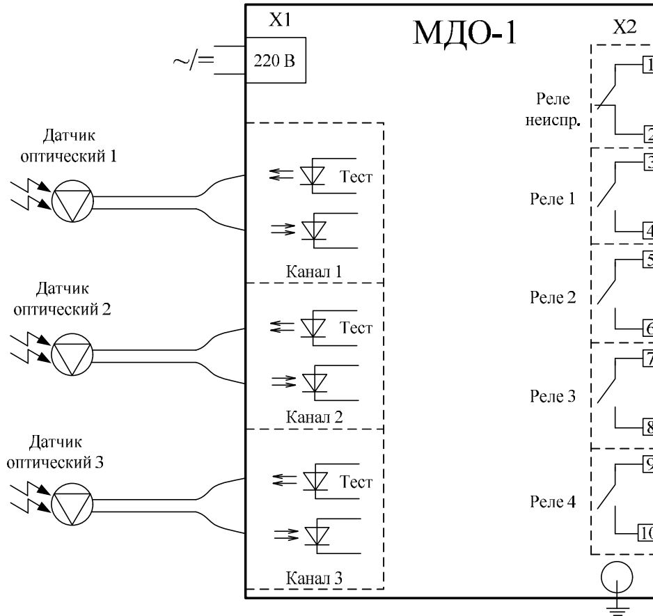
Рисунок В.1 – Схема подключения МДО-1
