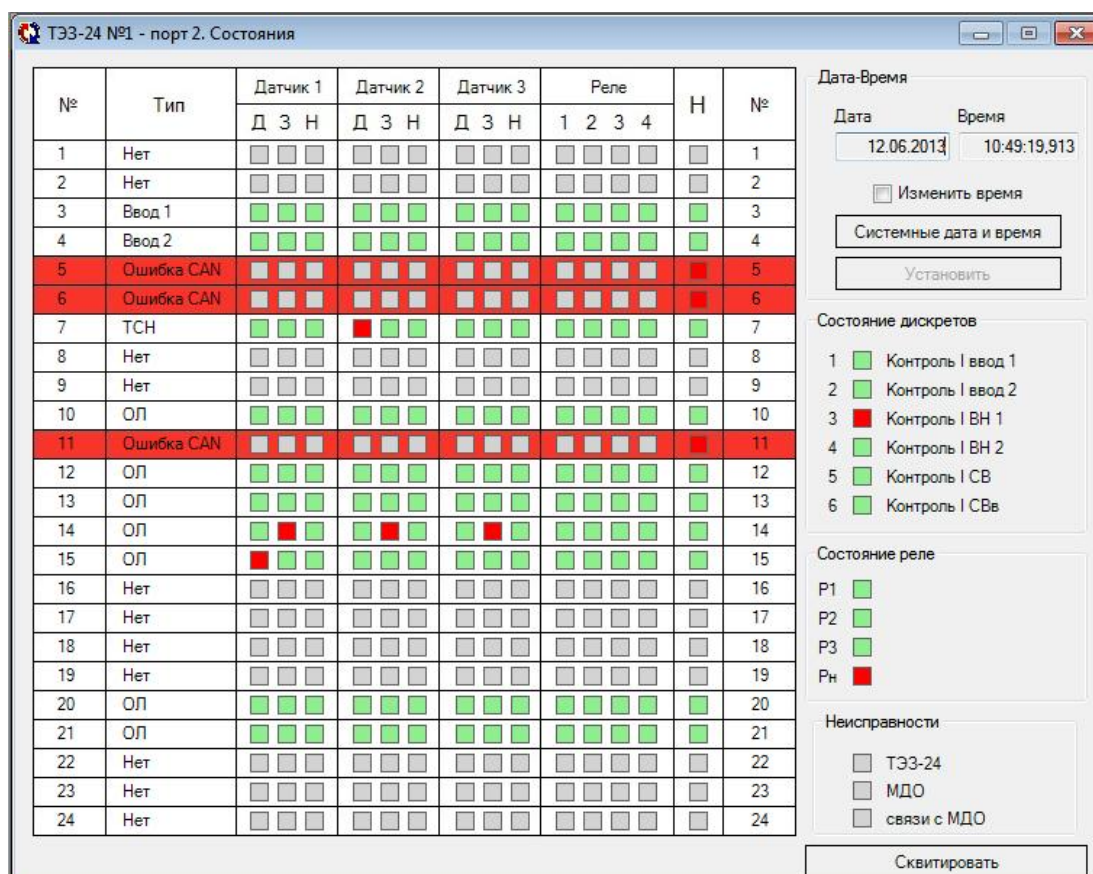
Рисунок 6.6 – Окно состояния ТЭЗ-24
