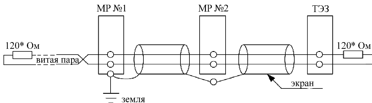
Рисунок 7.2 – Подключение кабеля
