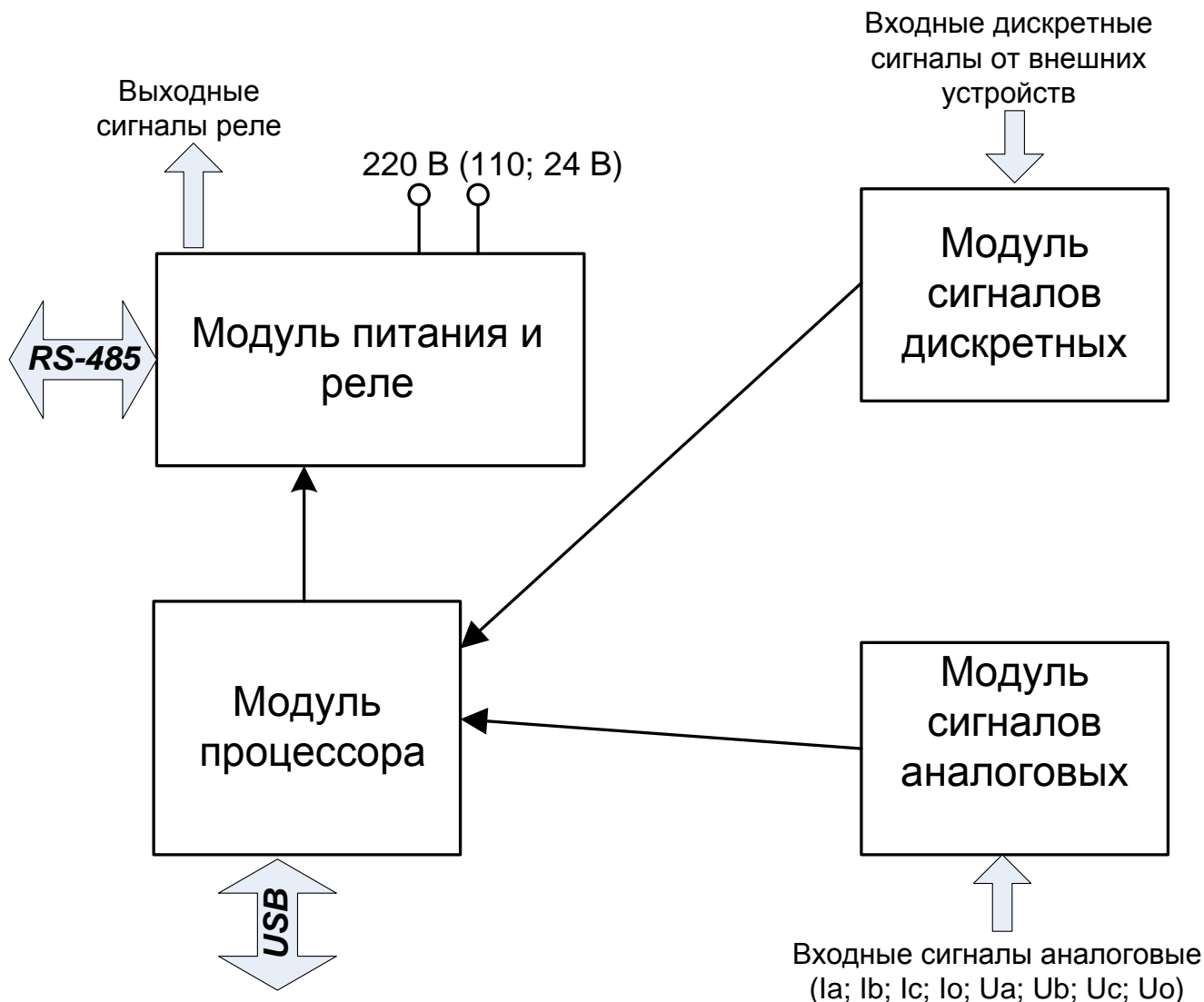
Рисунок 3.1 – Структура МР741
