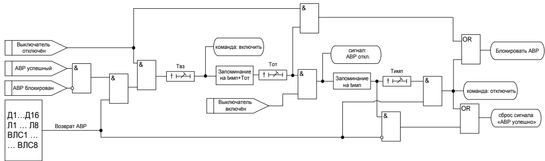
Рисунок 6.21 – Блок-схема логики возврата АВР
