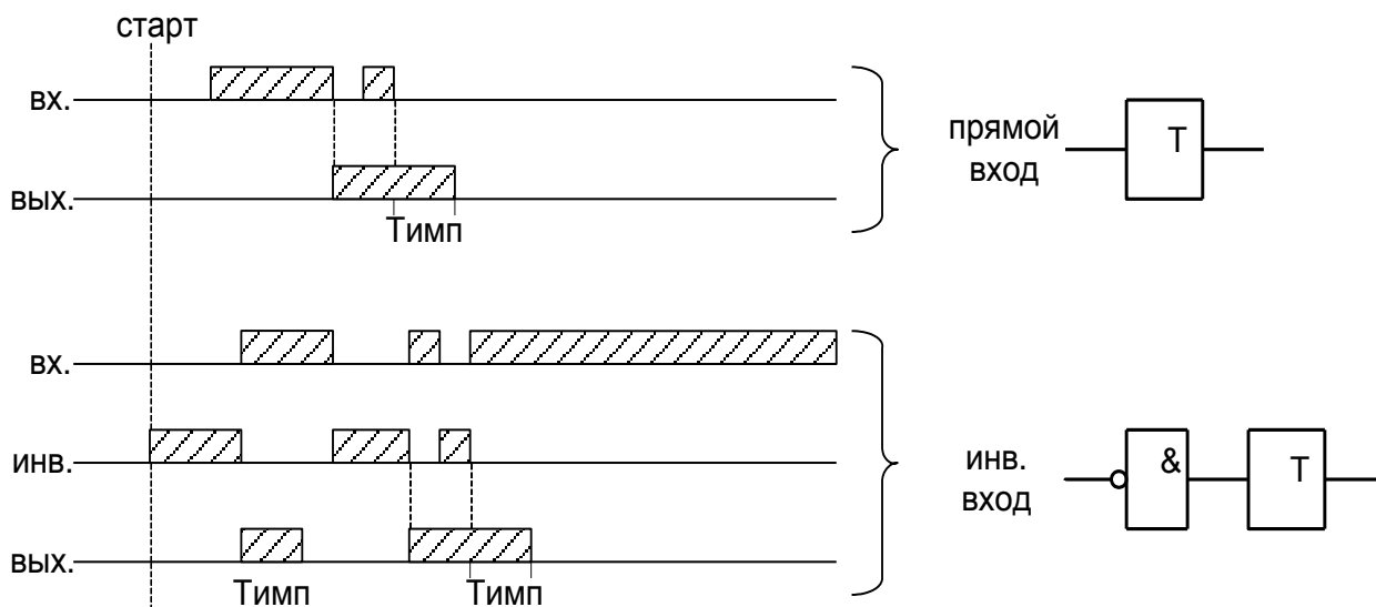
Рисунок 6.37 – Импульсный таймер по спаду типа 2 (таймер 6)
