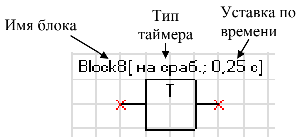
Рисунок 6.31 – Таймер
