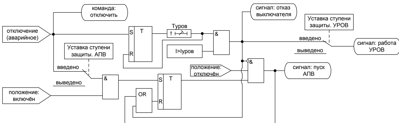
Рисунок 5.5 – Логика работы MP741 при аварийном отключении.
