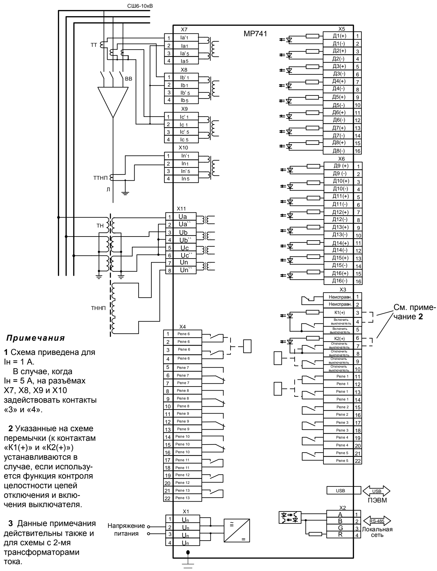
Схема с 3-мя трансформаторами тока (для I_n = 1 А)
