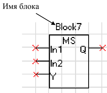
Рисунок 6.38 – Мультиплексор
