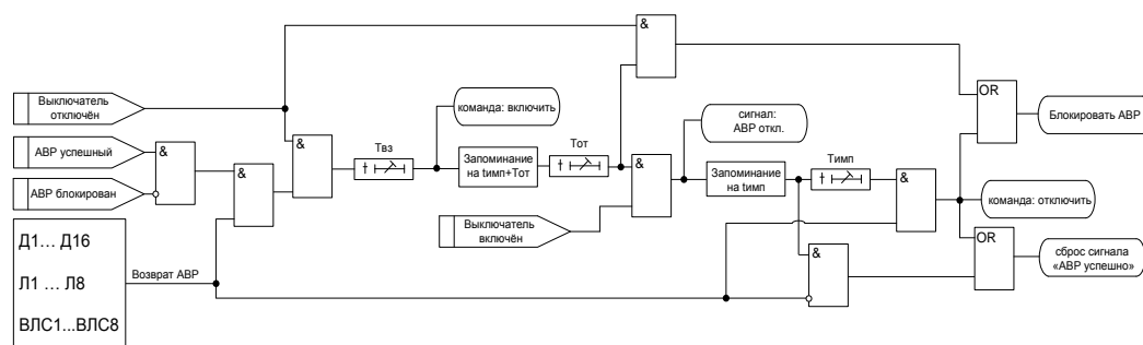
Рисунок 11.13 – Блок логики возврата АВР
