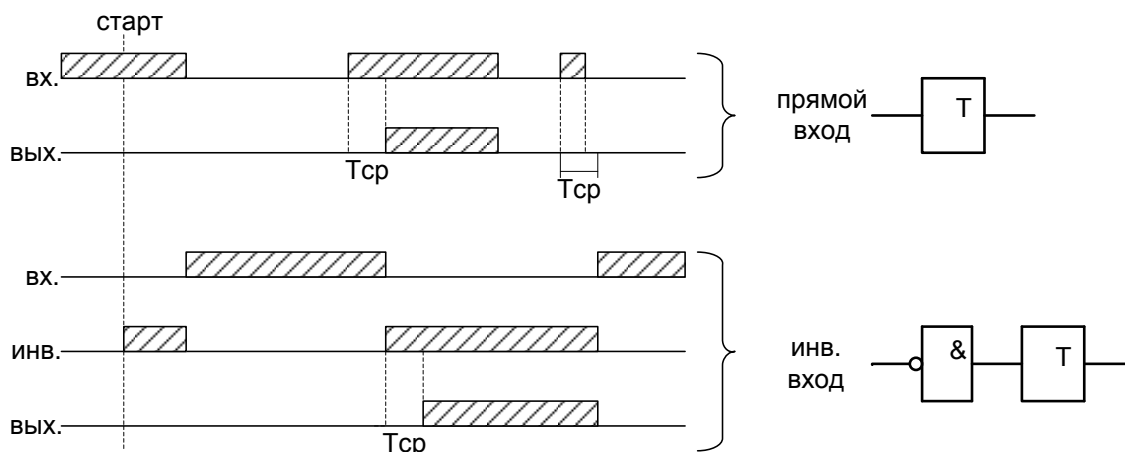
Рисунок 6.32 – Таймер на срабатывание (таймер 1)
