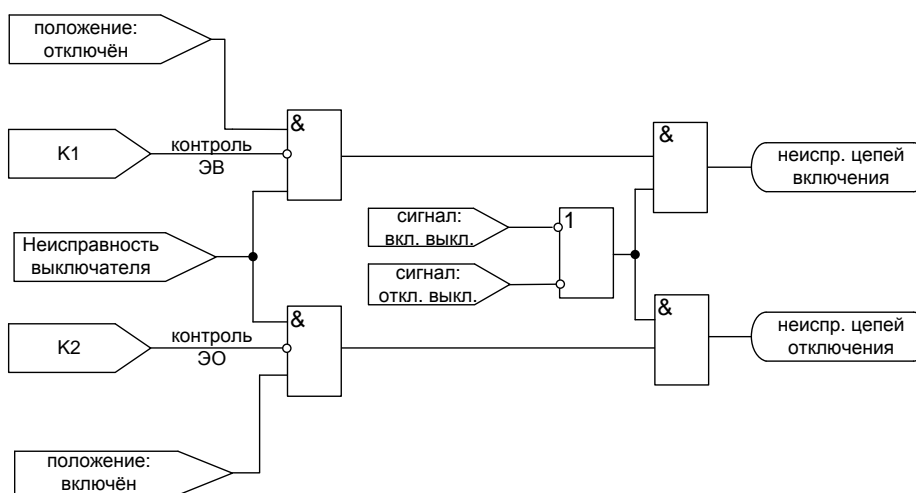
Рисунок 5.6 – Логическая схема контроля цепей управления
