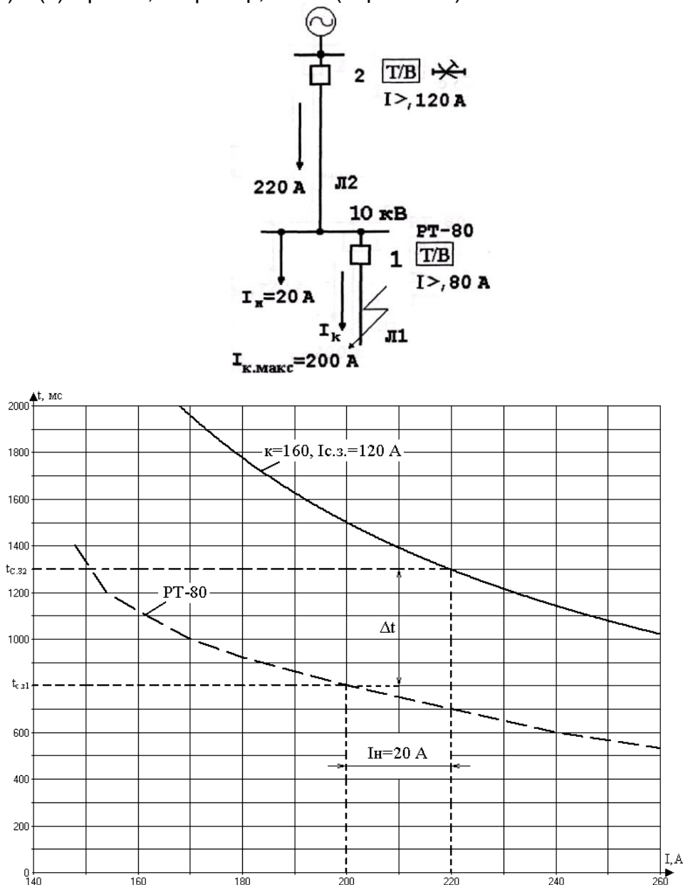
Рисунок 11.8 – Пример согласования характеристик устройств МР 700-й серии и дискового индукционного реле РТ-80
