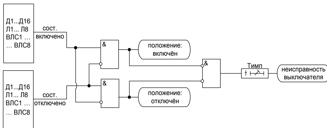
Рисунок 5.2 – Логика определения положения выключателя.
