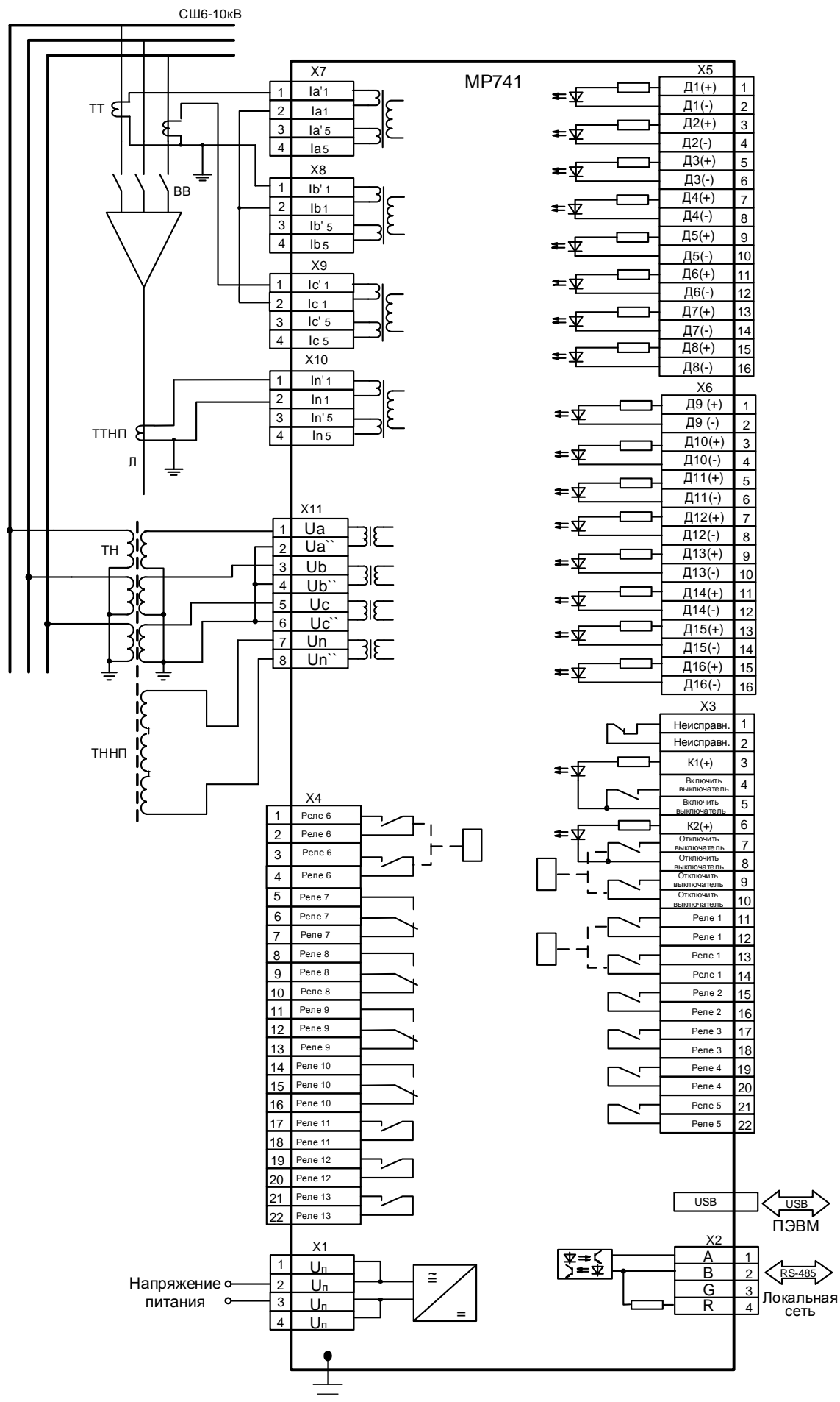
Схема с 2-мя трансформаторами тока (для I н = 1 А)
