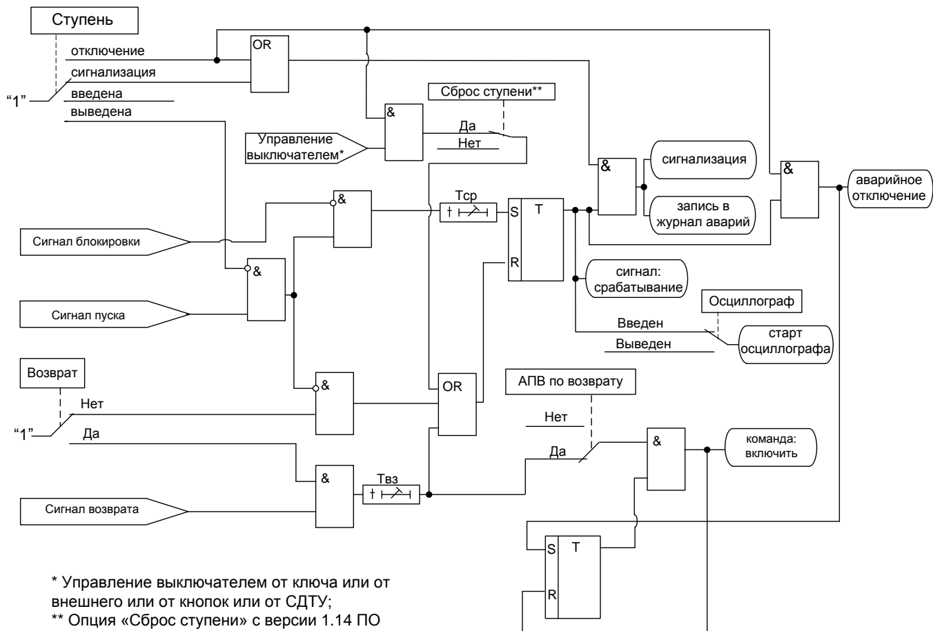
Рисунок 6.22 – Блок внешней защиты.
