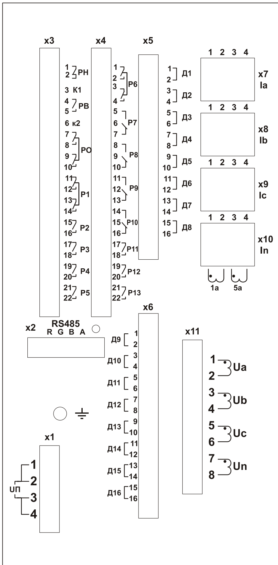
Вид задней панели MP741
