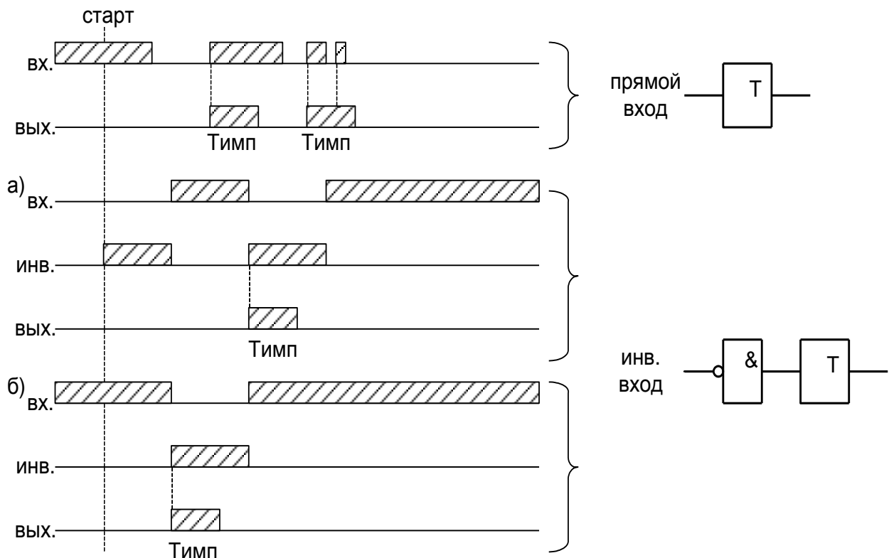
Рисунок 6.34 – Импульсный таймер по фронту типа 1 (таймер 3)
