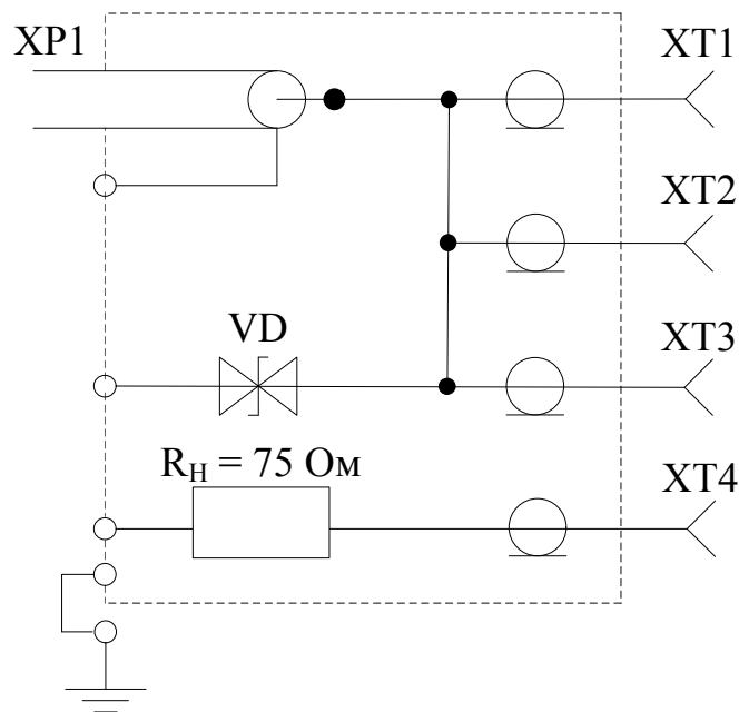
Рисунок 1.10 – Схема блока коммутации ВЧ соединений и нагрузки
