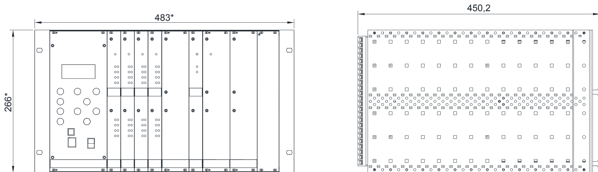
Рисунок А.1 – Передняя панель и вид сбоку СТРЕЛА М
