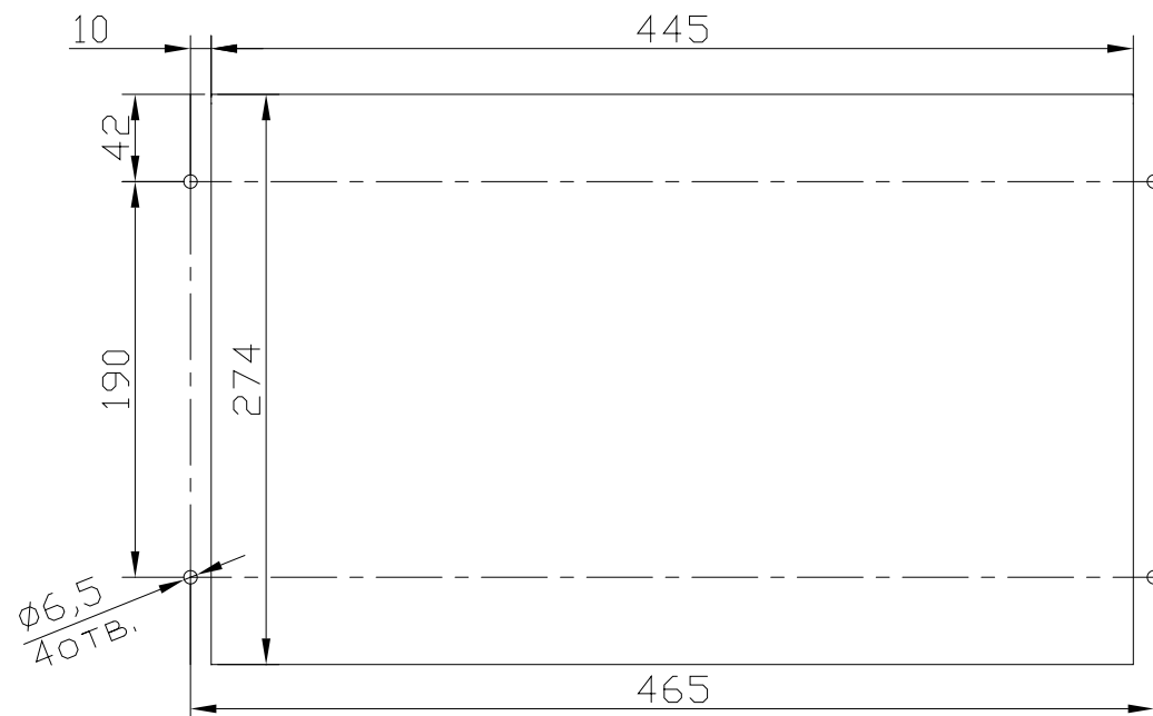
Рисунок А.3 – Размеры окна и монтажных отверстий под установку СТРЕЛА М
