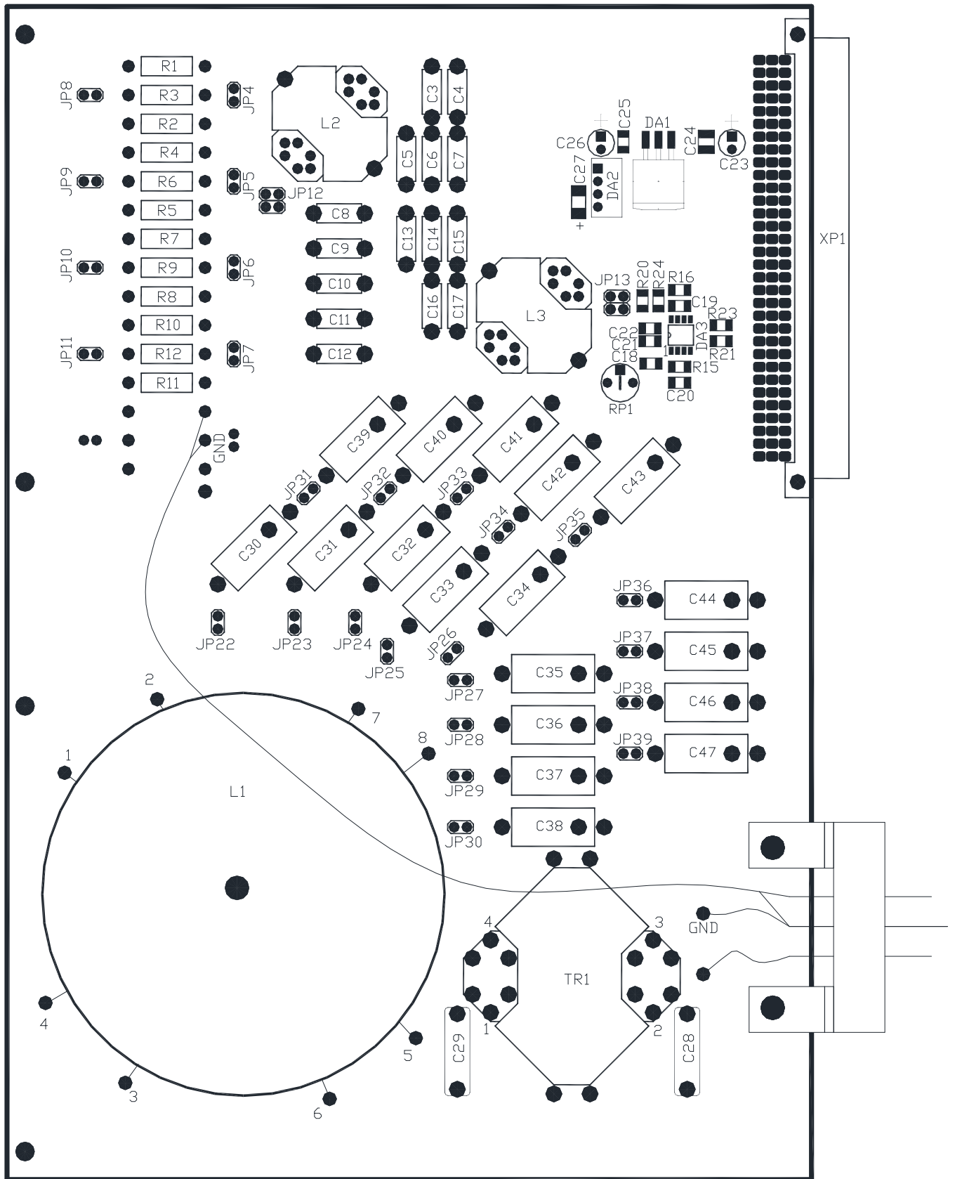
Рисунок 2.2 – Сборочный чертеж БФ
