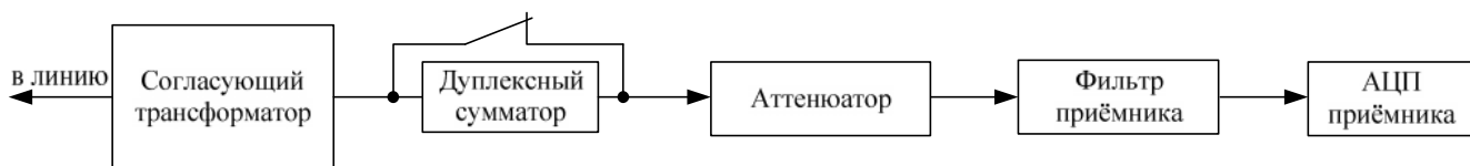
Рисунок 1.7 – Структурная схема приемного тракта в симплексном режиме работы
