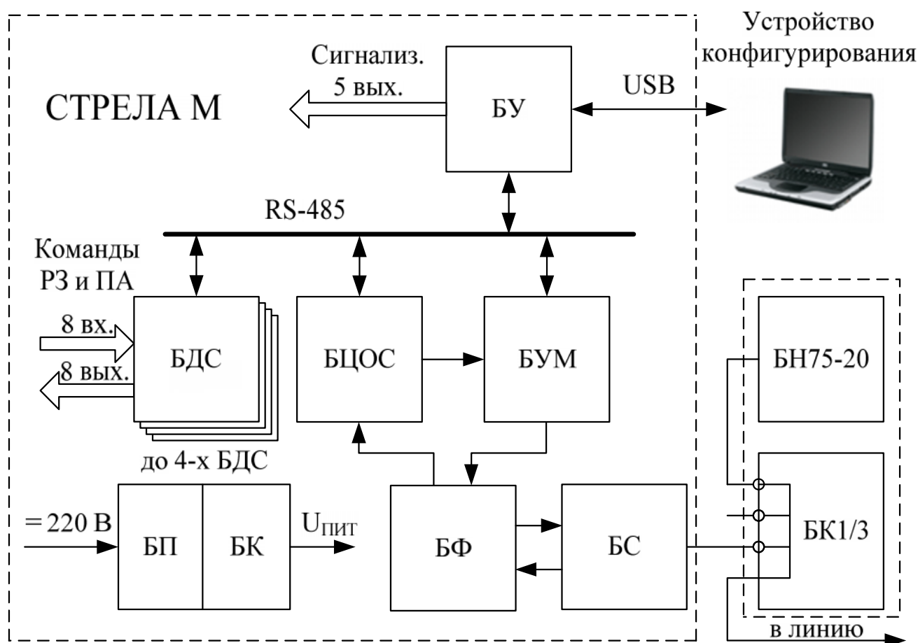
Рисунок 1.5 – Структурная схема СТРЕЛА
