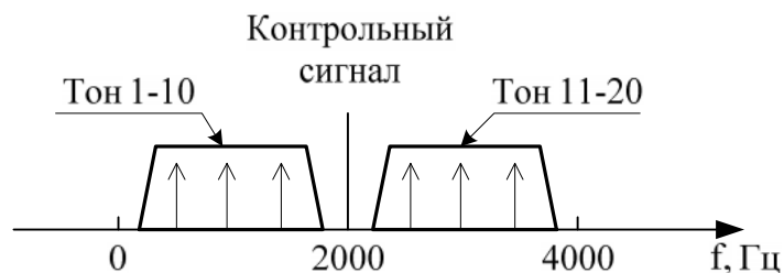
Рисунок 1.3 – Частотный план канала
