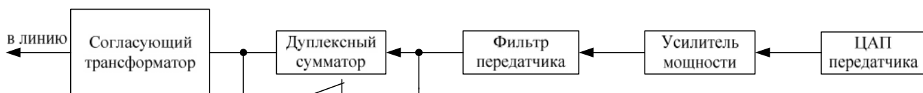
Рисунок 1.8 – Структурная схема передающего тракта в симплексном режиме работы
