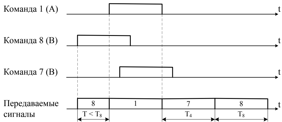
Рисунок 1.30 – Комплексная передача параллельных и последовательных команд
