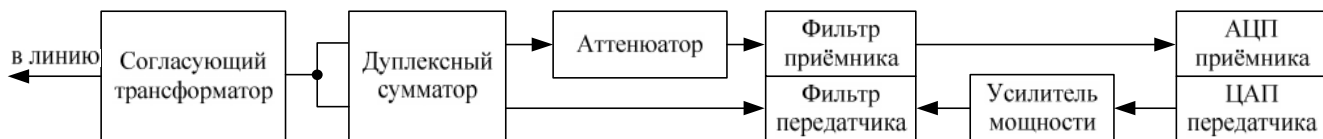
Рисунок 1.6 – Структурная схема ВЧ тракта аппаратуры СТРЕЛА в дуплексном режиме работы
